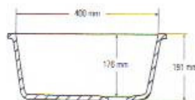
Sección lateral
