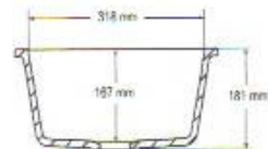
Sección lateral
